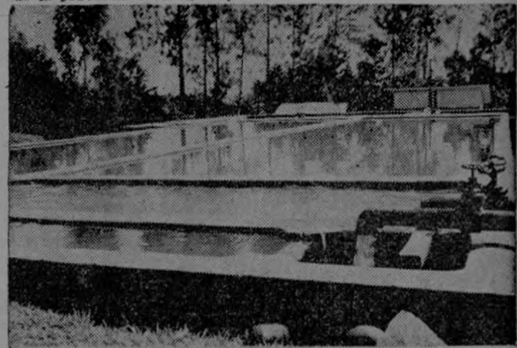
A pesar de que el caudal de agua que llega de las fuentes es mínimo, la planta no está capacitada para procesar por el sistema de filtros lentos, ni siquiera 11 litros por segundo, lo que agrava más la crítica situación que se atraviesa en Palmares por la falta de agua en toda la ciudad.
